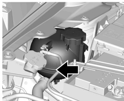
Tanque de compensación de refrigerante del motor 1.3L I3
